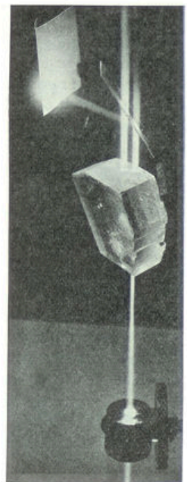
Hoe een lichtstraal door een kalkspaatkristal in tweeën wordt gedeeld en één der beide uit-tredende stralen door een stuk glas niet teruggekaatst wordt. — Illustratie uit: „Het wonder van het Licht.“
