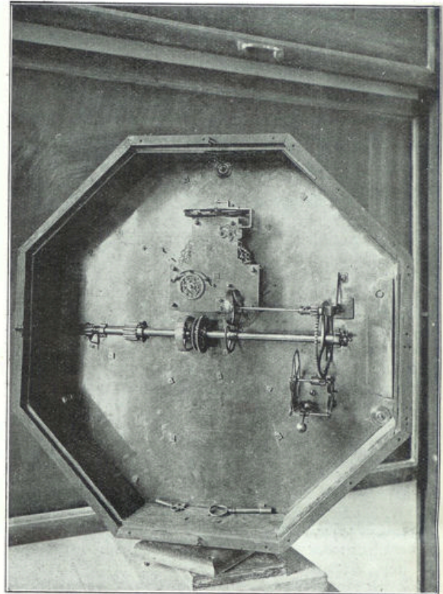
Achterzijde van het planetarium, in 1682 door den Haagschen uurwerkmaker Johannes van Ceulen gemaakt volgens berekeningen en aanwijzingen van Huygens.
