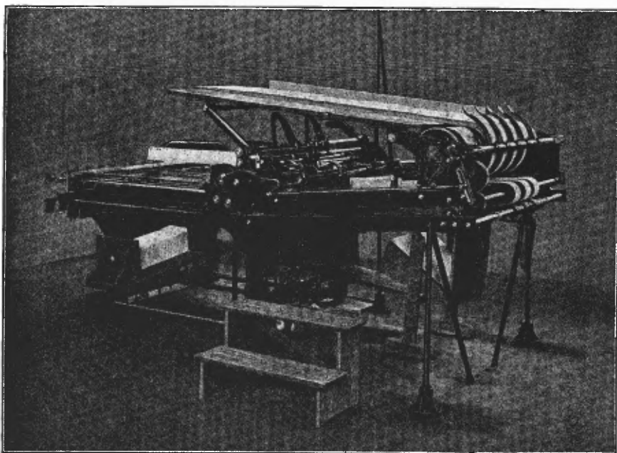
Vouwmachine met automatischen inleg.
