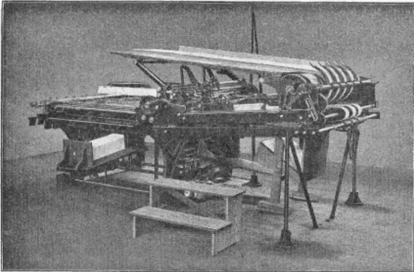
Vouwmaschine met automatischen inleg.
