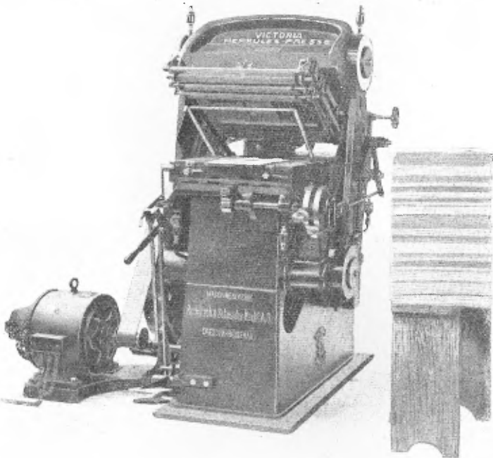
Stempelpers met electro-motor.
