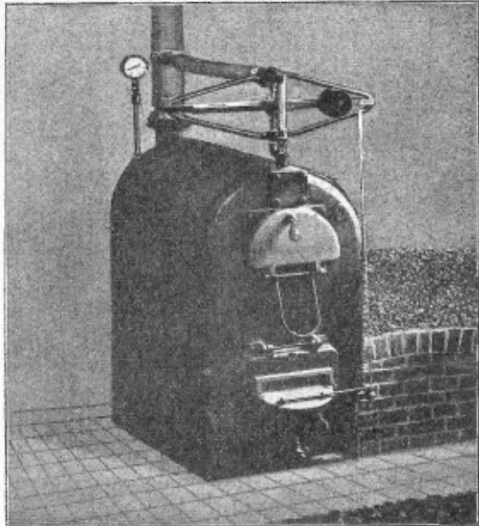
Ketel van de centrale-verwarming.
